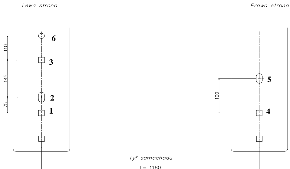
Rys. 2 . Widok ramy samochodu (od spodu)
